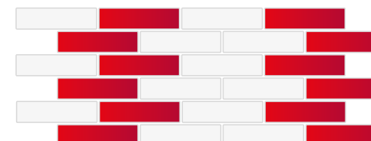
WIĄZANIE WOZÓWKOWE PRZESUNIĘCIE O 1/2 CEGŁY
