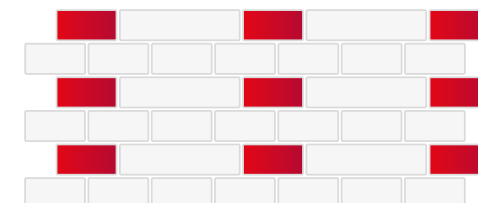
WIĄZANIE HOLENDERSKIE
