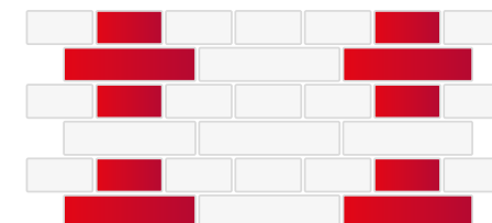
WIĄZANIE KRZYŻOWE TYP 1
